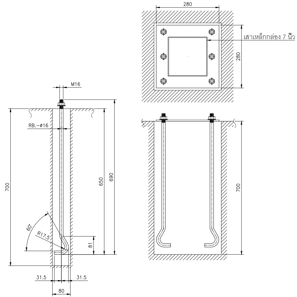
แบบขยาย ตอมอ เส้า หน้าเป็นบาสฯ
